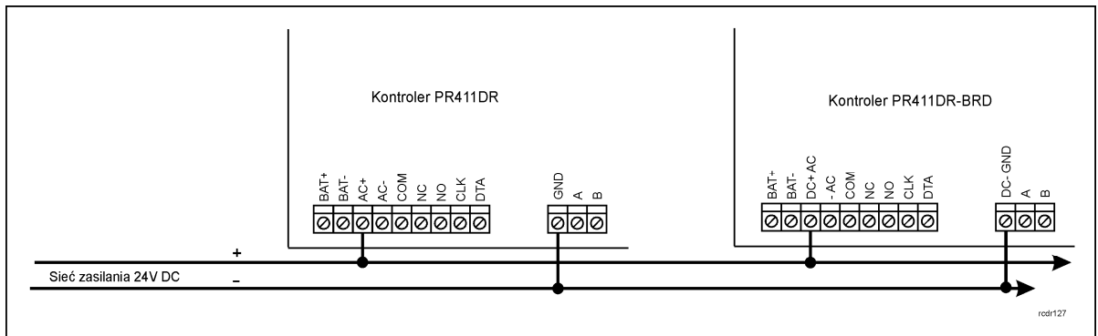
Rys. 7 Zasilanie kontrolerów PR411DR z sieci prądu stałego 24VDC
