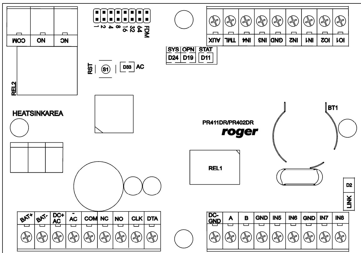
Rys. 2 Kontroler PR411DR-BRD
