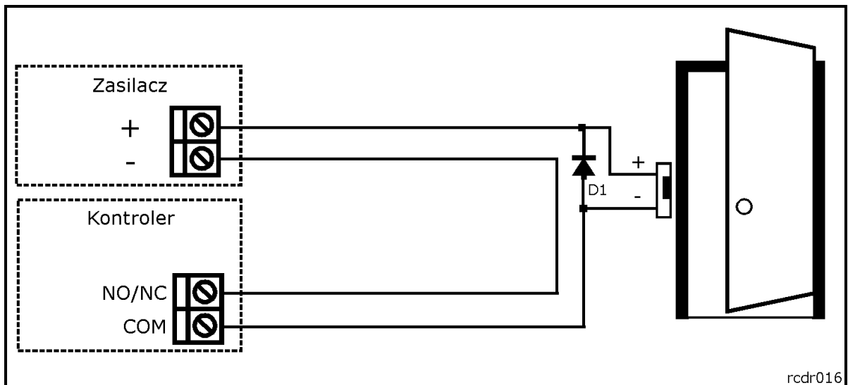
Rys. 8 Podłączenie elementu wykonawczego
