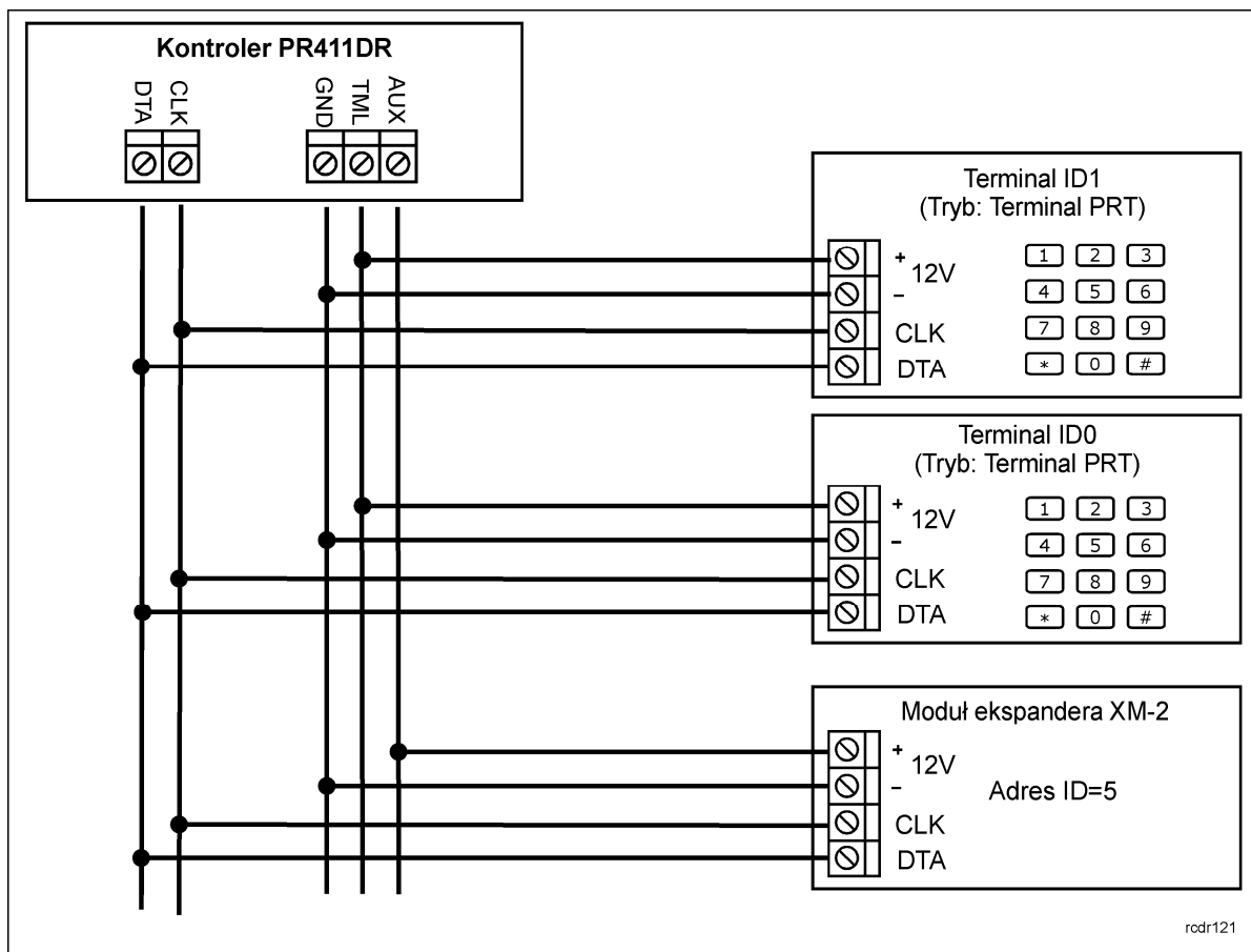
Rys. 9 Sposób podłączenia czytników serii PRT oraz modułu XM-2 do PR411DR
