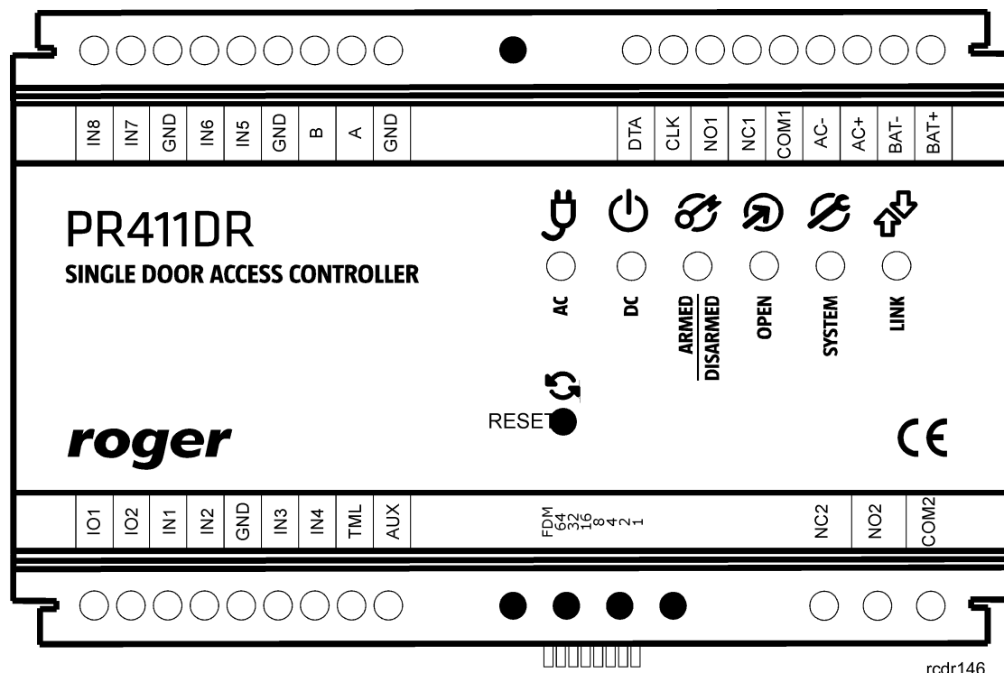
Rys. 1 Kontroler PR411DR
